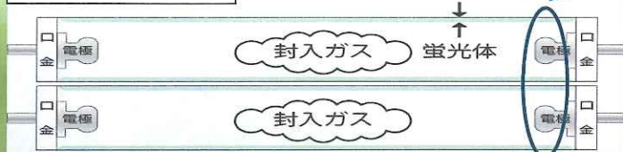
CCFL 管の構造図
