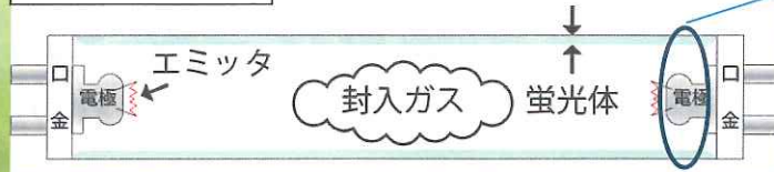
蛍光灯の構造図
