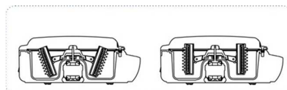
水平ローターの動作図
